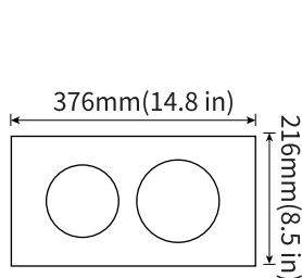
Płyta wentylacyjna
