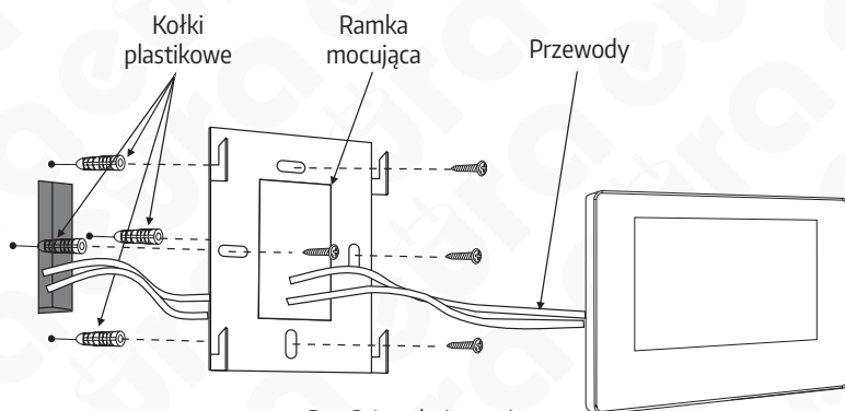
Rys. 2. Instalacja monitora
