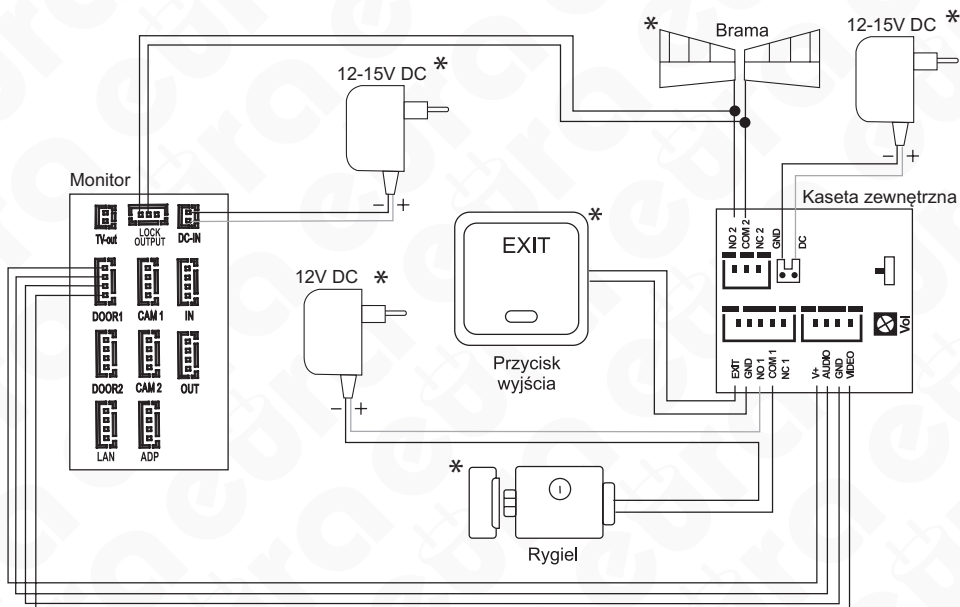
Rys. 4. Schemat połączeniowy z wykorzystaniem zasilaczy sieciowych
