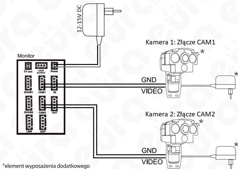
Rys. 7. Schemat podłączenia dodatkowych kamer
