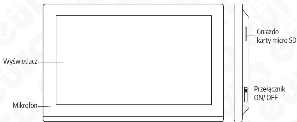
Rys. 1. Budowa monitora
