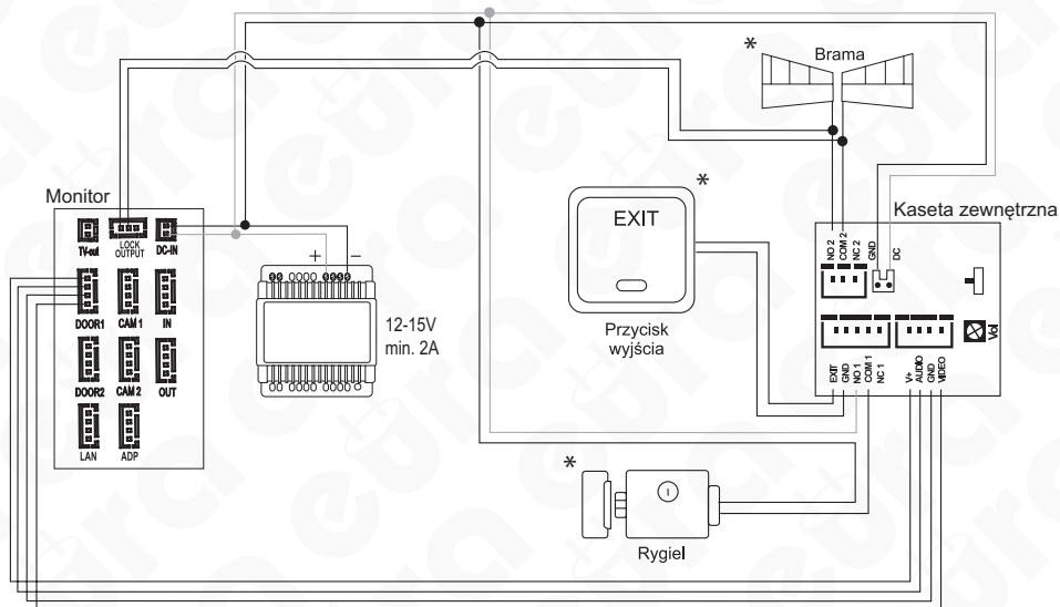
Rys. 5. Schemat podłączenia z wykorzystaniem jednego zasilacza
