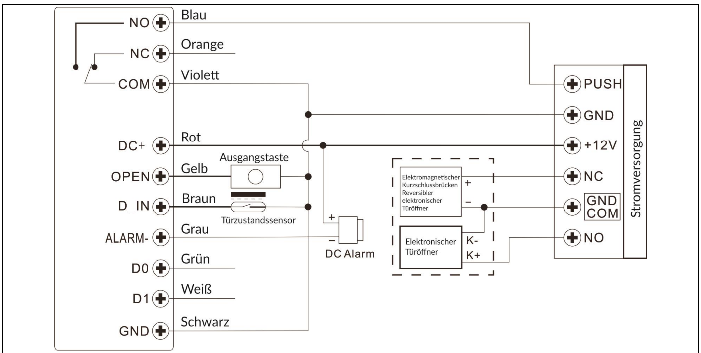
Abb. 2 Zusätzlicher Schaltplan
