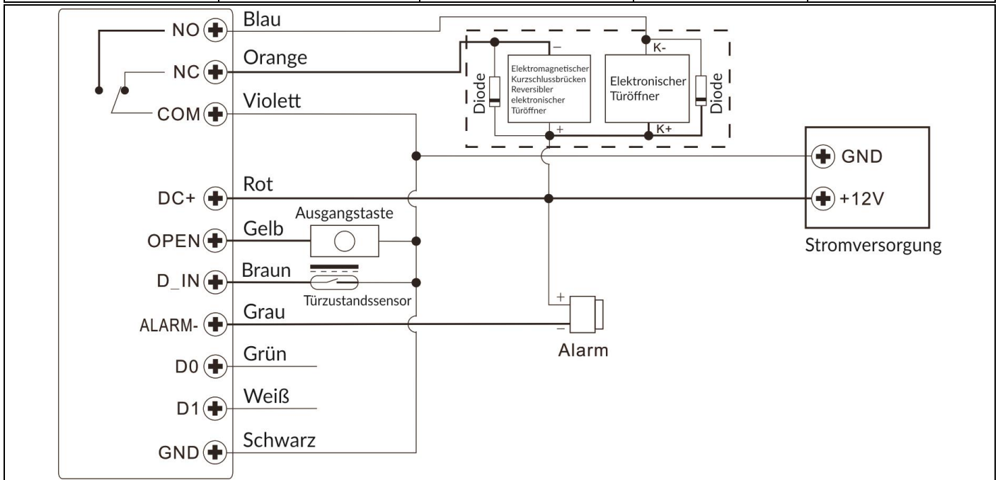
Abb. 1 Standard Schaltplan
